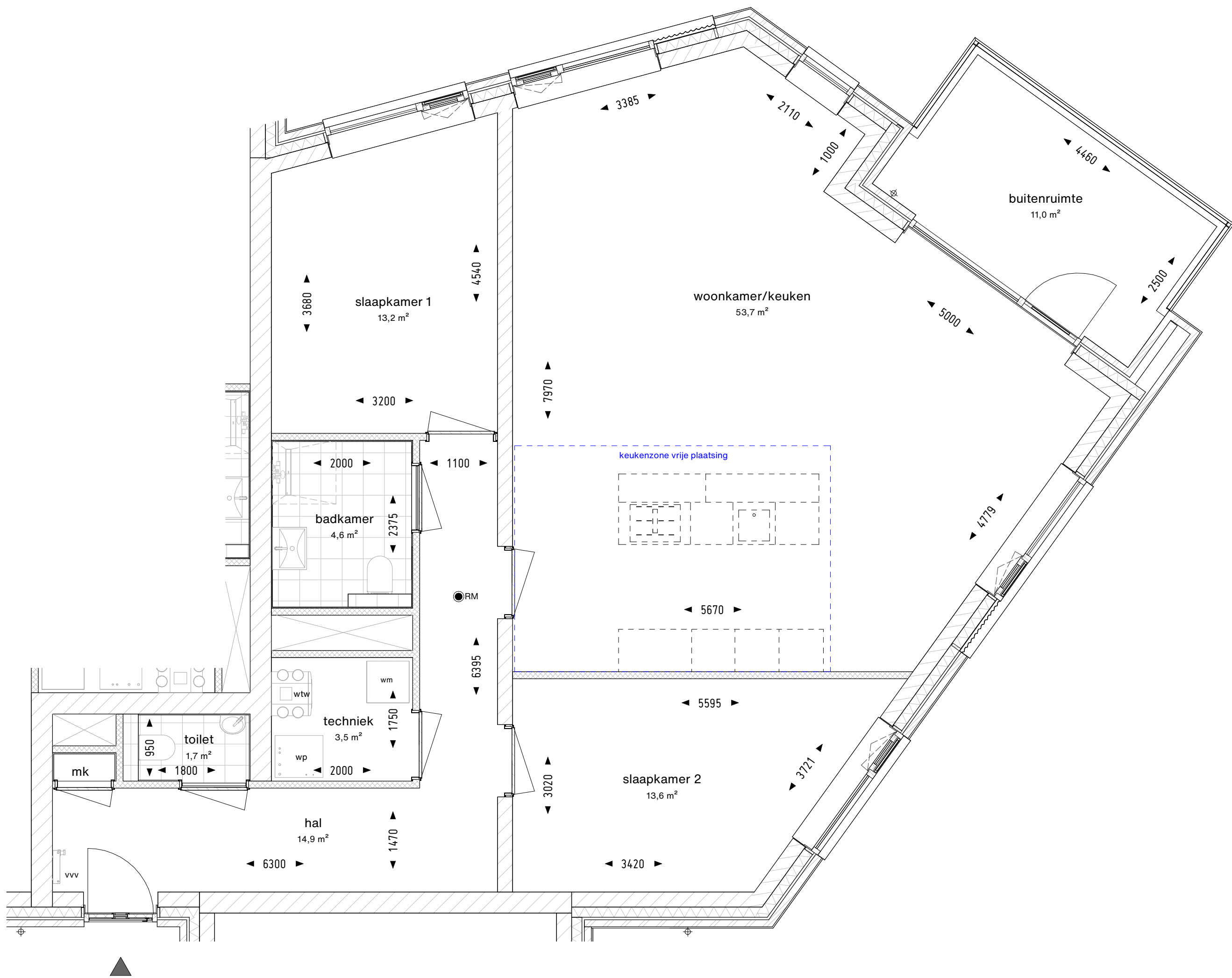
Type D - bnr 15 - 24, 1e en 2e verd. 1 : 50
