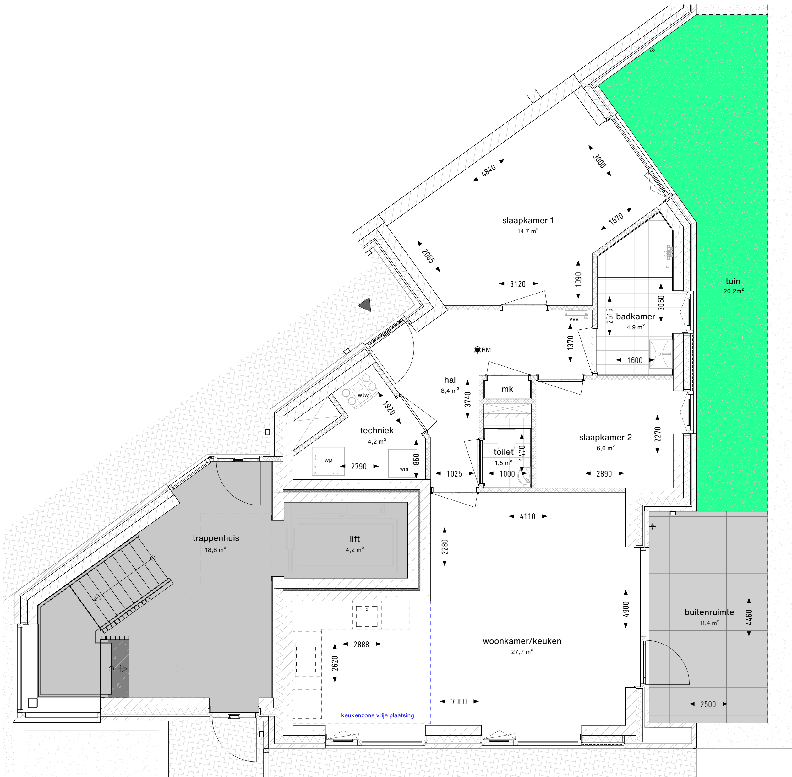
Type E - bnr 07, begane grond 1 : 50
