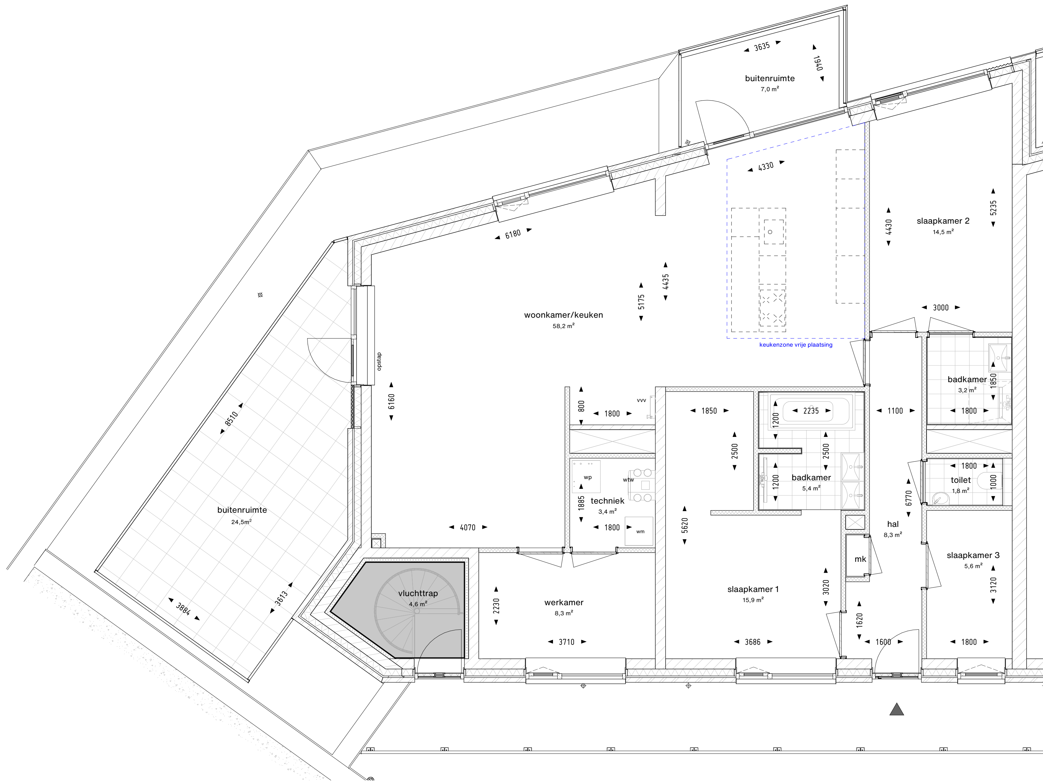
Type I - bnr 26, 3e verd. 1 : 50
